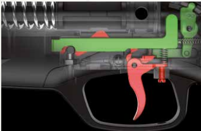
XT trigger with adjustable first stage travel XT-Abzug mit justierbarem Vorzugsweg
