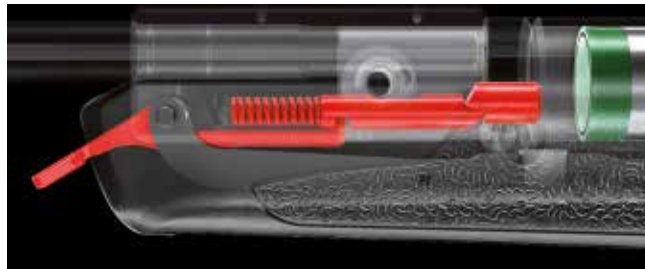
The wedge lock ensures a snug barrel fit – form-fit and force-fit barrel lock for consistent precision Passgenaue Lauflagerung durch Keilverriegelung – form- und kraftschlüssig, wiederholbar präzise
