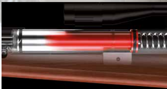
The rotary piston absorbs the torsion forces of the spring Der Drehkolben schluckt die Torsionskräfte der Feder
